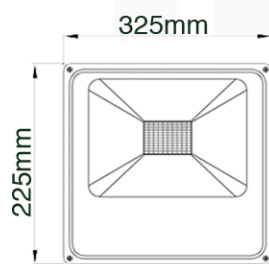
ALZADO FRONTAL
