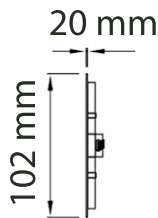
ALZADO LATERAL
