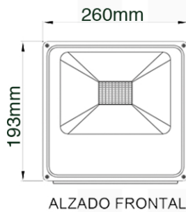
ALZADO FRONTAL
