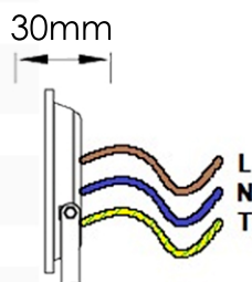
ALZADO LATERAL
