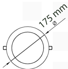
ALZADO FRONTAL
